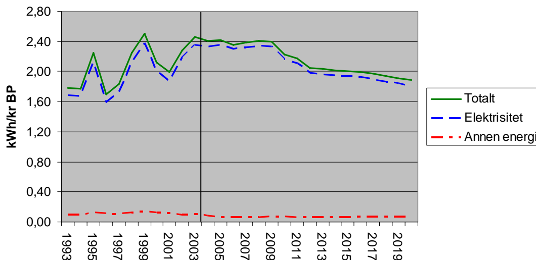
Figur 4.17: Historisk og framskrevet energiintensitet for næringen ikke jernholdige metaller, basert på B1.
